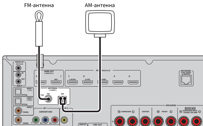
Аппарат (вид сзади)
