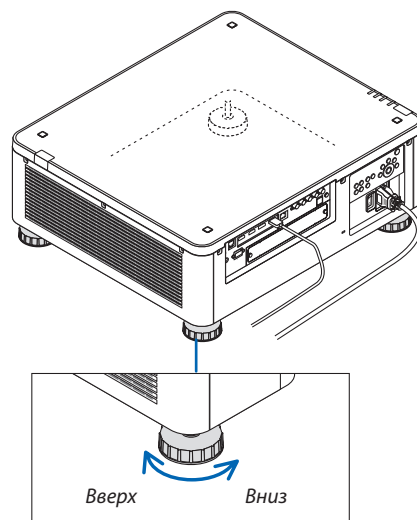
Ножка для регулирования наклона (есть еще одна сзади)
